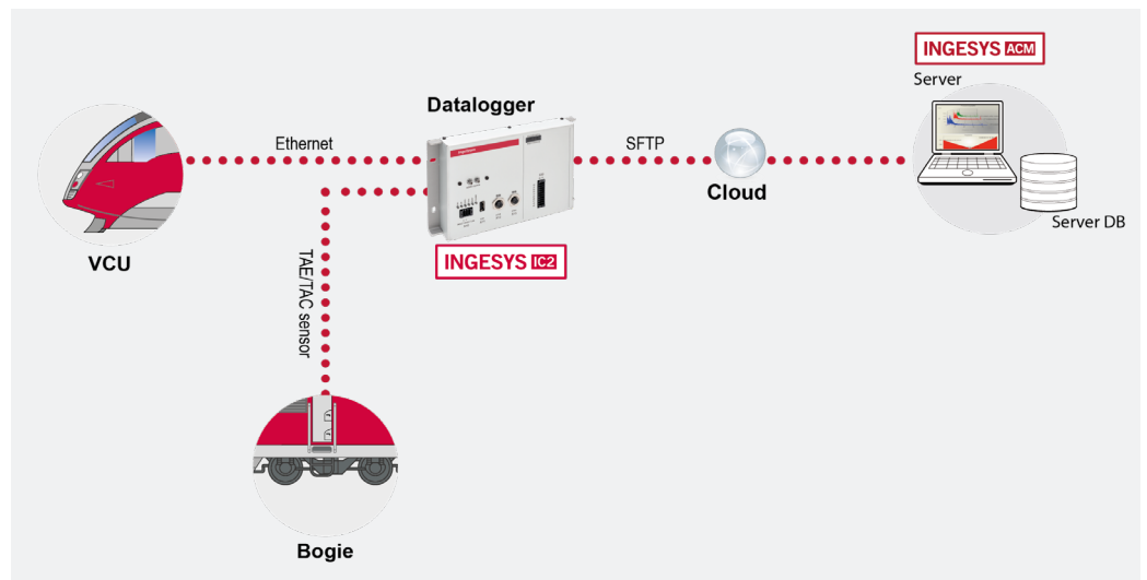
Ejemplo de solución RCM de Ingeteam para el sector ferroviario
