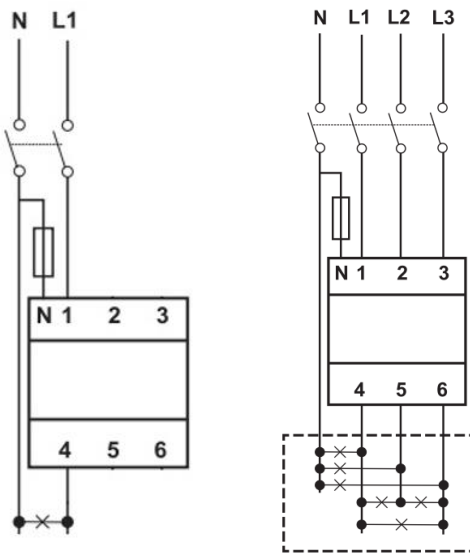
Installation monophasée
